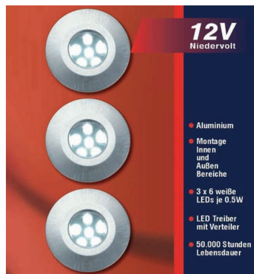
DI 61037 LED-Einbauset / LED-Set IP65, Aluminium / aluminium, rund / round 3x 6LED/12V/0,5W; weiß / white Ø 40mm, Tiefe / depth 57mm
