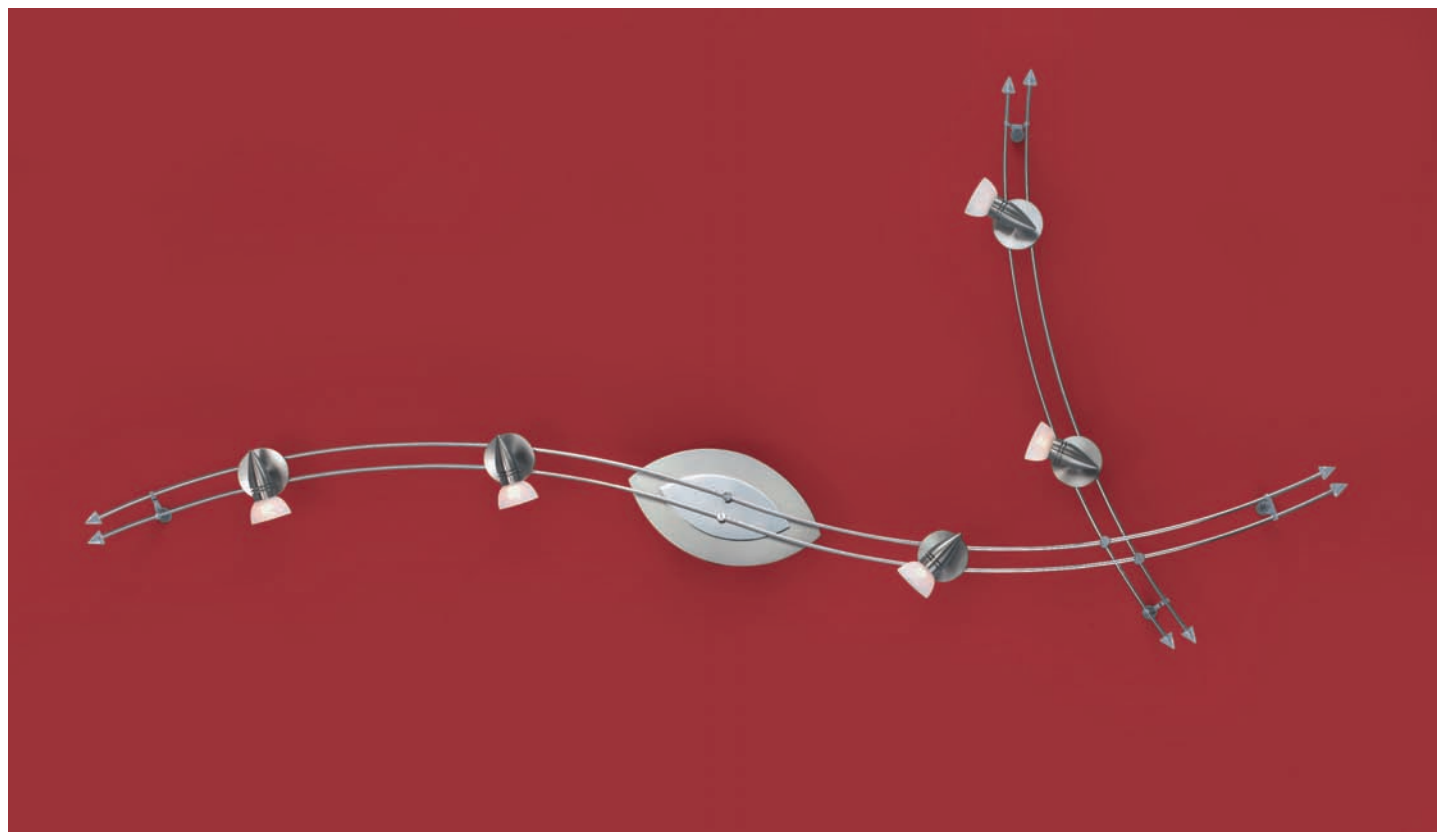
WO 9156.05.64.5440 Nickel matt / Nickel matt finished 5x GY6,35/12V/35W Länge 200 cm, Breite 100 cm
