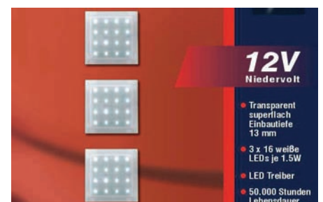
DI 61035 LED-Einbauset / LED-Set IP20, Kunststoff / Plastic, quadratisch / quadratic 3x 16LED/12V/1,5W; weiß / white 70x70x13mm
