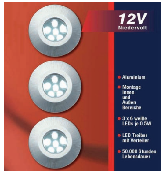
DI 61037 LED-Einbauset / LED-Set IP65, Aluminium / aluminium, rund / round 3x 6LED/12V/0,5W; weiß / white Ø 40mm, Tiefe / depth 57mm
