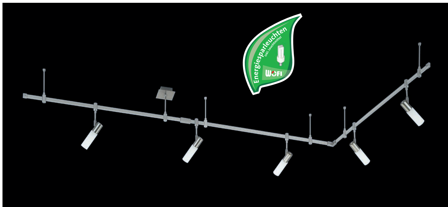
WO 9754.05.64.5210 Nickel matt / Nickel matt finished 5x E14/230V/8W – incl. ESL Länge 300 cm
