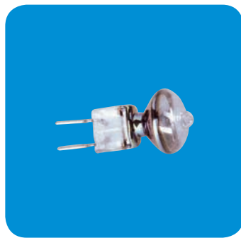
LA 512335 Halogen Mini Reflektor / halogen mini reflector warm weiß / warm white, 2700K 12V G6,35/35W, 30°
