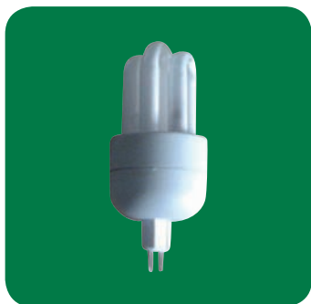
CAL 571310 Energie Sparlampe Mini / energy saving lamp mini warm weiß / warm white 2700K 230V G9/5W
