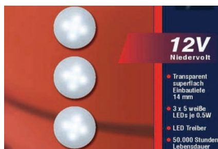
DI 61034 LED-Einbauset / LED-Set IP20, Kunststoff / Plastic, rund / round 3x 5LED/12V/0,5W; weiß / white Ø 50mm, Höhe / high 14mm
