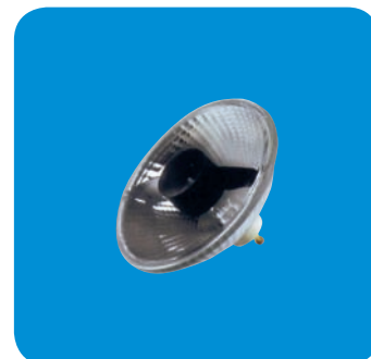
LA 575652 Halogen-Leuchtmittel / halogen lamp ES 111 warm weiß / warm white, 2700K 230V GU10/50W, 24°, Ø 11,1cm
