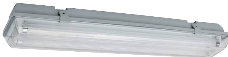
DI 50061 2x 18W Leuchtstoffröhre / fluorescent lamp IP65, Polycarbonate Diffuser Länge 650mm, Breite 116mm, Höhe 87mm Bestellmenge/Pieces in the box: 6 Stücke / 6 pieces mit Leuchtstoffröhre / incl. fluorescent lamp 58 Watt Daylight 6500 K
