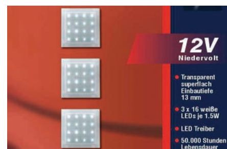
DI 61035 LED-Einbauset / LED-Set IP20, Kunststoff / Plastic, quadratisch / quadratic 3x 16LED/12V/1,5W; weiß / white 70x70x13mm
