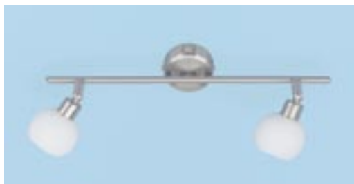
2 x G 9, 40W Breite ca. 32 cm WO 7790.02.64.0000 Nickel-matt, Nickel, matt finished mit Schalter
