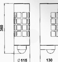
AL 690209 IP 44, A 60, max. 75 W, E 27 Opal glas mit Bewegungsmelder (BWM)
