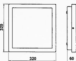
AL 696133 IP 54, 3 x TC 11 W, G 23 Opal Scheibenglas
