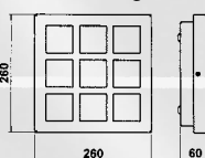
AL 696134 IP 54, 2 x TC 9 W, G 23 Opal Scheibenglas
