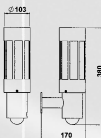
AL 690241 IP 44, A 60, max. 75 W, E 27 Opal glas mit Bewegungsmelder (BWM)
